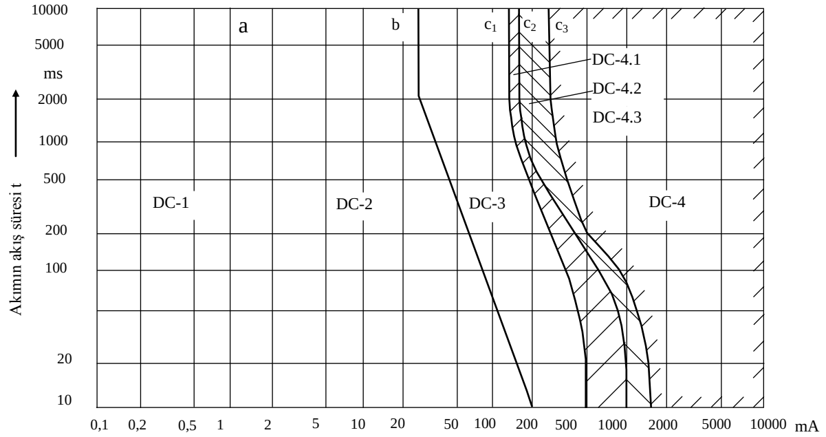
Şekil-C.4 Doğru akım etkilerinin akım/zaman bölgeleri
